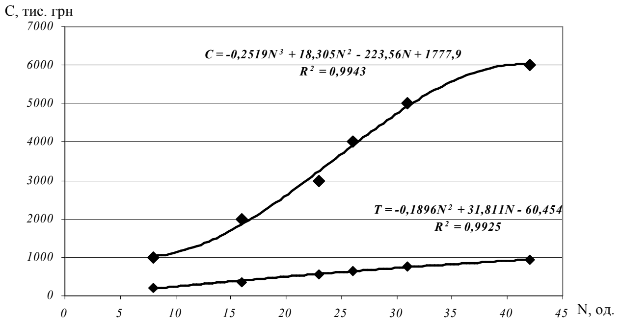
Рисунок 3 - Залежність достовірності показників надійності та економічності від витрат на випробування
