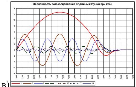
Рисунок 6 – Залежність коефіцієнтів Фур'є від довжини котушки шляхової структури
