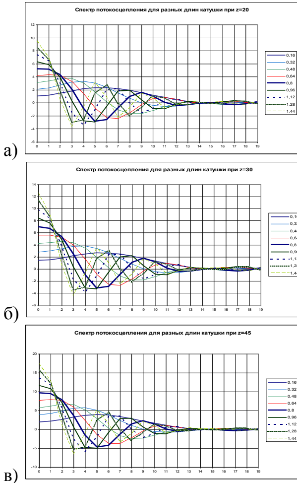
Рисунок 7 – Залежність коефіцієнтів ряду Фур'є для різних довжин катушки шляхової структури від номера гармоніки
