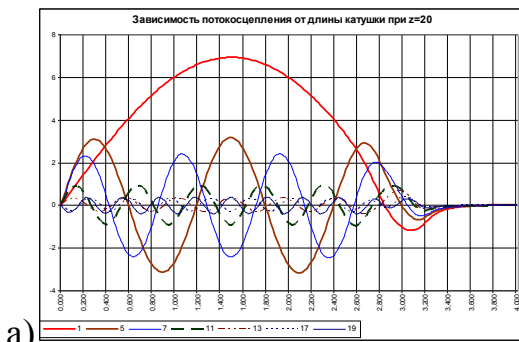
Рисунок 5 – Залежності потокозчеплення котушки шляхової структури з блоком постійних магнітів від їх взаємного зміщення
