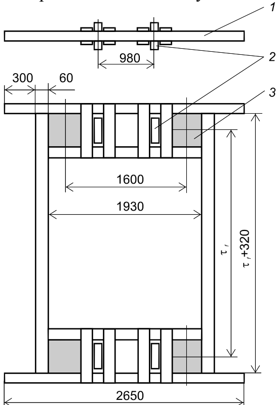
Рисунок 9 – Експериментальний візок
