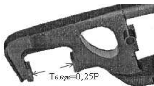
Схема 5 – Навантаження на буксові прорізи по черзі
