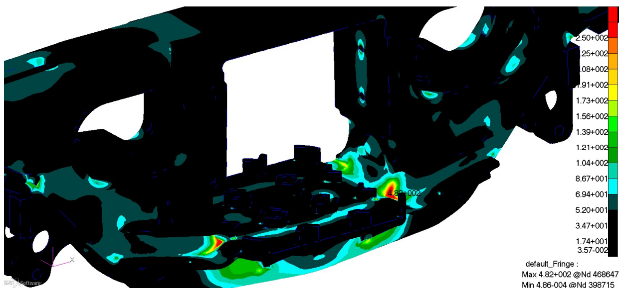
Рисунок Є.1 – Розподіл еквівалентних напружень в нижньому кутку центрального ресорного прорізу з внутрішньої сторони, МПа (I розрахунковий режим).
