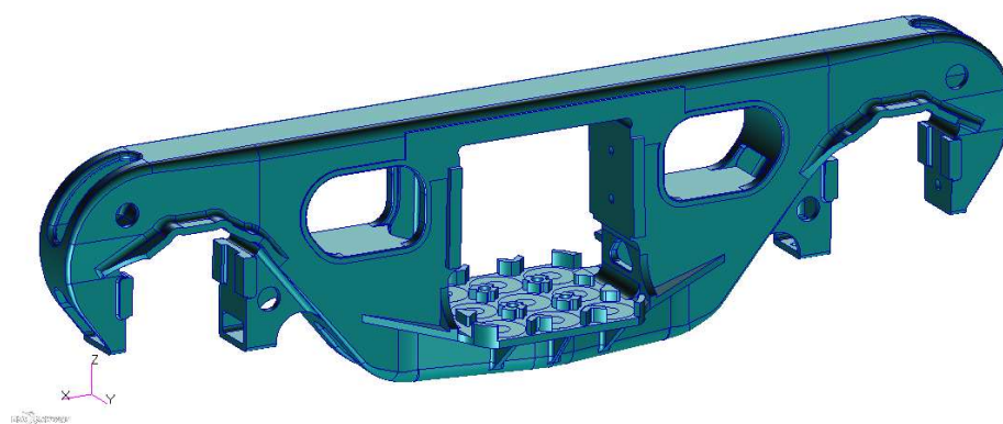
Рисунок 2.1 – Геометрична модель бічної рами
