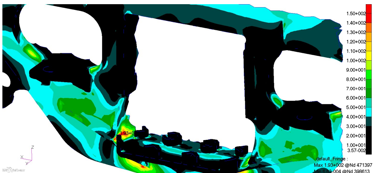
Рисунок Є.2 – Розподіл еквівалентних напружень в нижньому кутку центрального ресорного прорізу із зовнішньої сторони, МПа (III розрахунковий режим).
