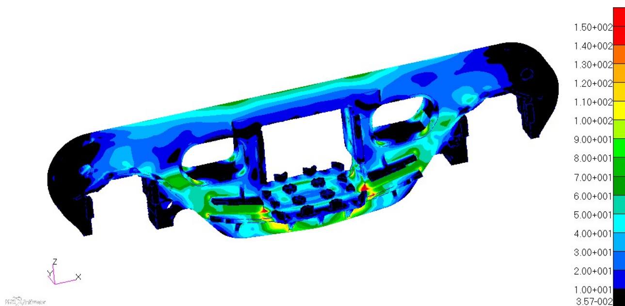
Рисунок Б.5 – Розподіл еквівалентних напружень в бічній рамі, варіант навантаження \partial , МПа.
