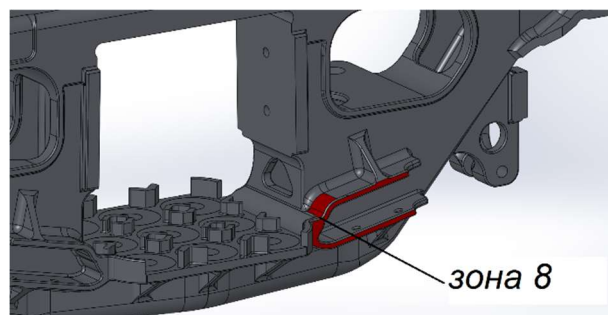
Рисунок 5.8 – Зона підсилення поличок для триангеля
